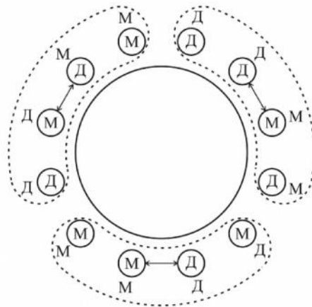
СЛИКА 3. Лема 1 - За n = 6 потребни се 3 чекори.
