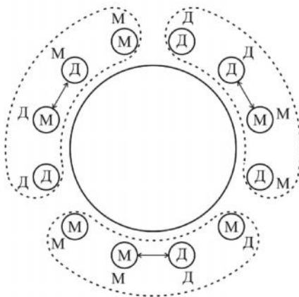
Слика 1. Лема 1 - За n = 6 потребни се 3 чекори.
