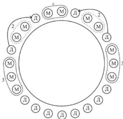
Слика 2. Лема 2 - Во групите заокружени со \cdots\cdots има вкупно 4 момчиња, а во групите заокружени со ---- има вкупно 8 момчиња. При оваа конфигурација, за n = 12 и 4 осамени девојчиња, имаме решение во 4 чекори.
