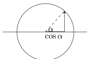
Slika 7: Trisekcija kuta s trigonometrijskog aspekta
