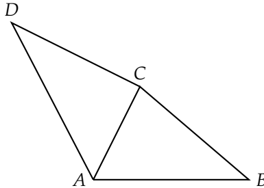
Slika 9. Euklidov dokaz obrata Pitagorinog poučka
